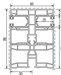
Führungsschiene PVC Doppelführung
