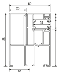
Führungsschiene ALU Einzelführung
