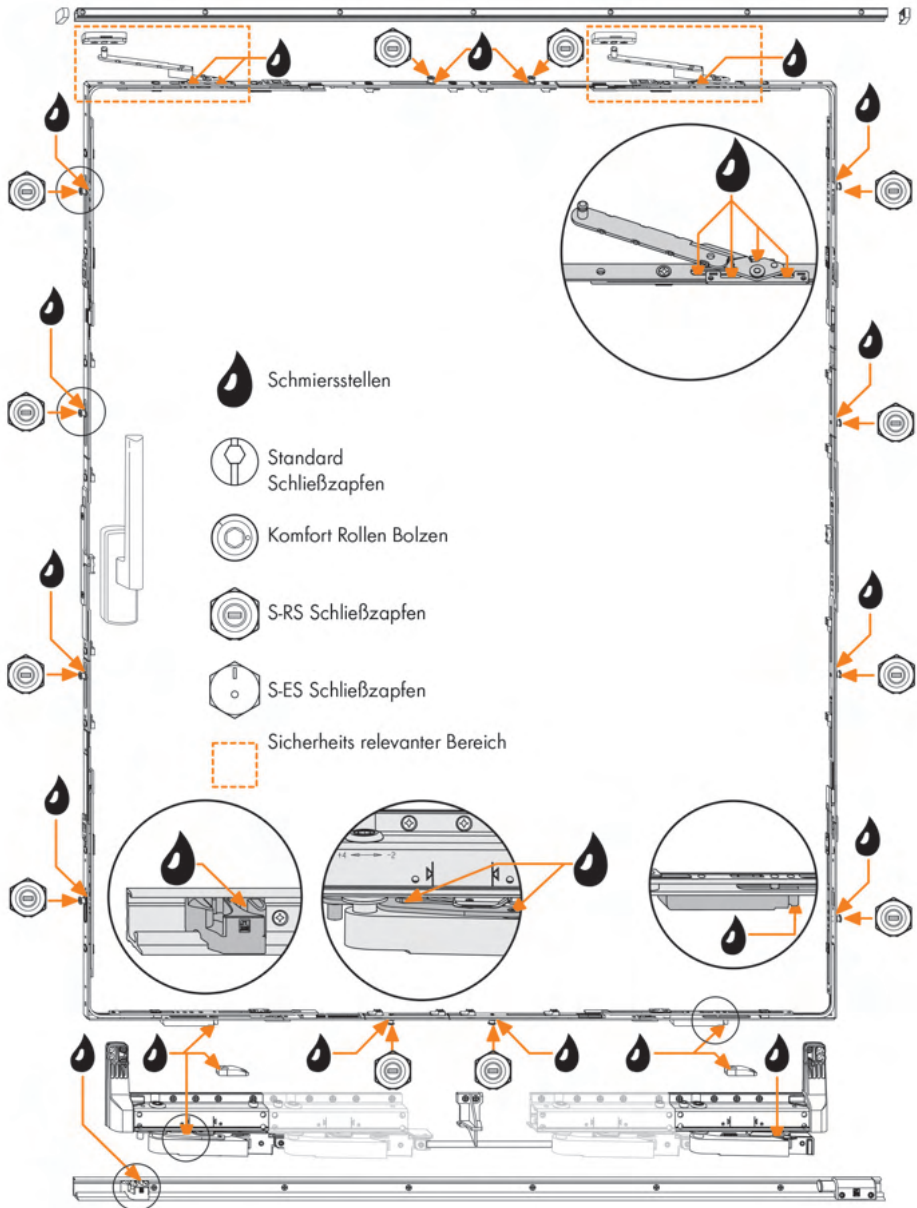
Abbildung zeigt den Parrallel-Schiebe-Kipp-Beschlag PSK 200-Z PLUS Der vorhandene Zentralverschluss kann abweichen!
