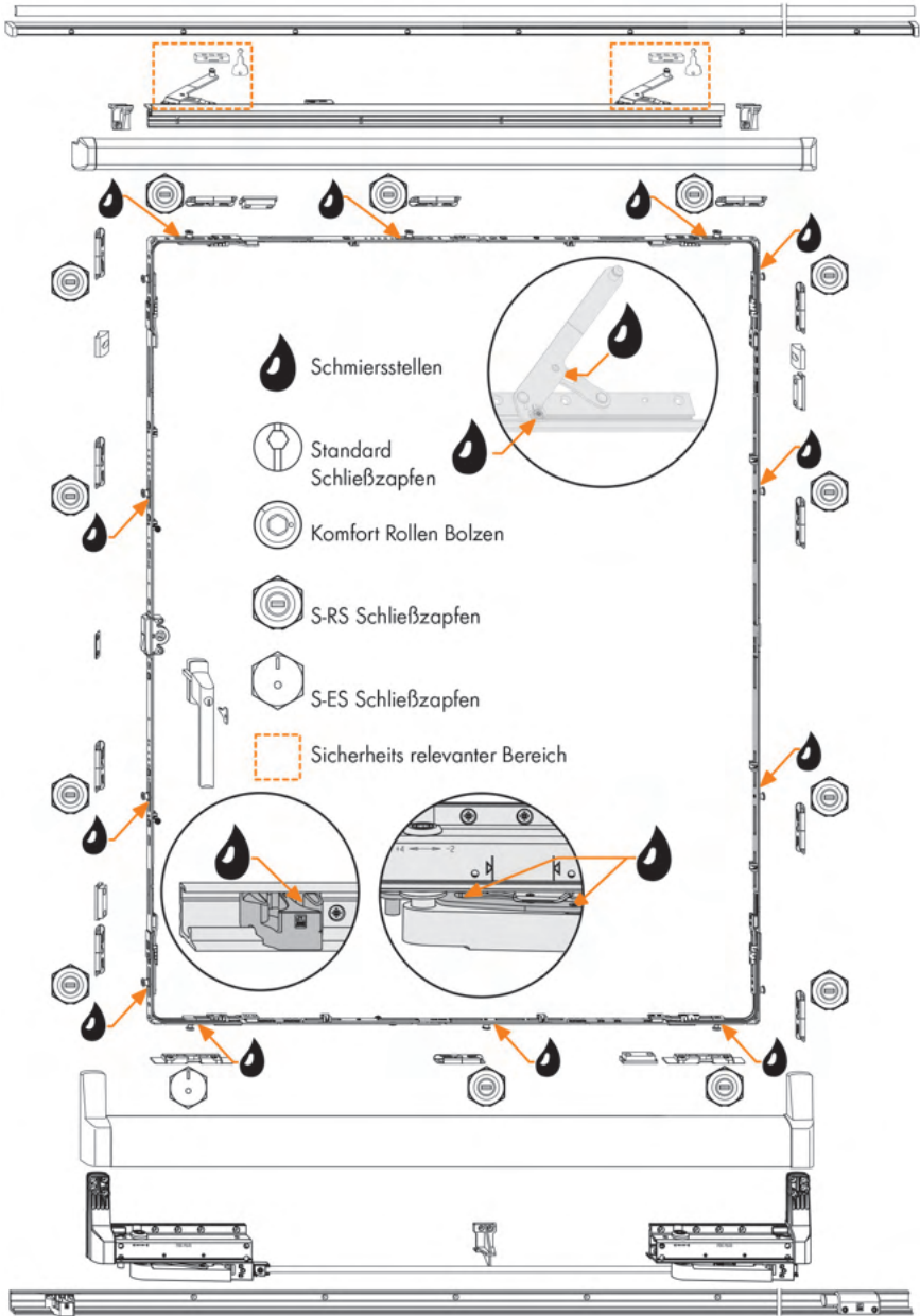
Abbildung zeigt den Parrallel-Schiebe-Kipp-Beschlag PSK 160 PLUS Der vorhandene Zentralverschluss kann abweichen!
