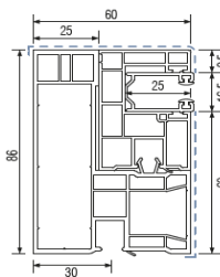
Führungsschiene PVC Einzelführung
