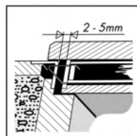
Schließblech/Stulp Abstand 2 bis 5 mm.
