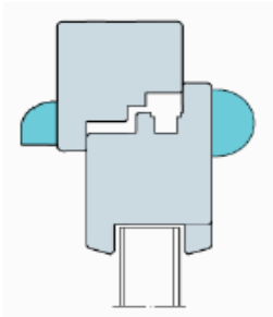
Einbau in Rahmen und Flügel
