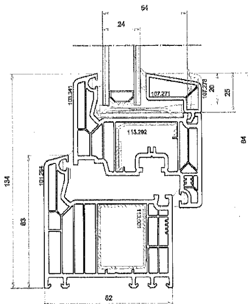
Bild 2 Schnitte des Systems SOFTLINE 76
