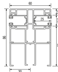
Führungsschiene ALU Einzelführung
